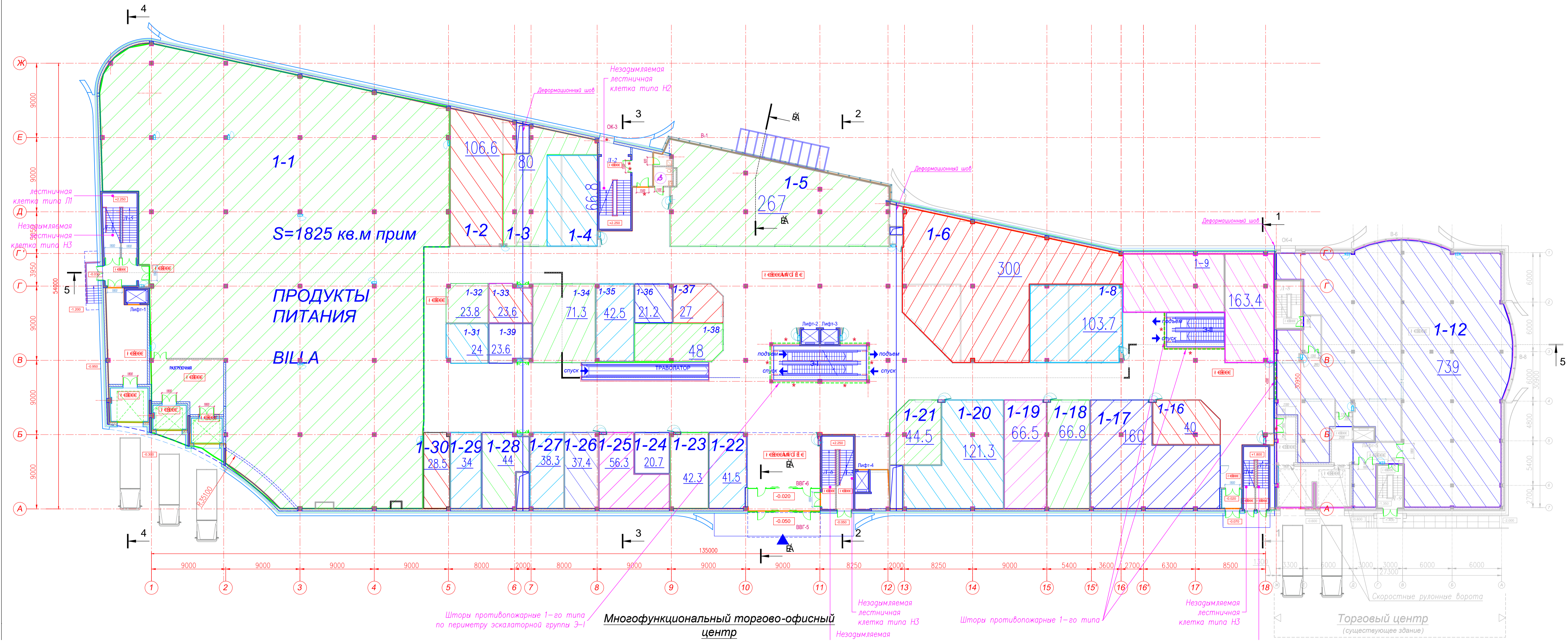
План первого этажа на отм. ±0.000 масштаб 1:200
